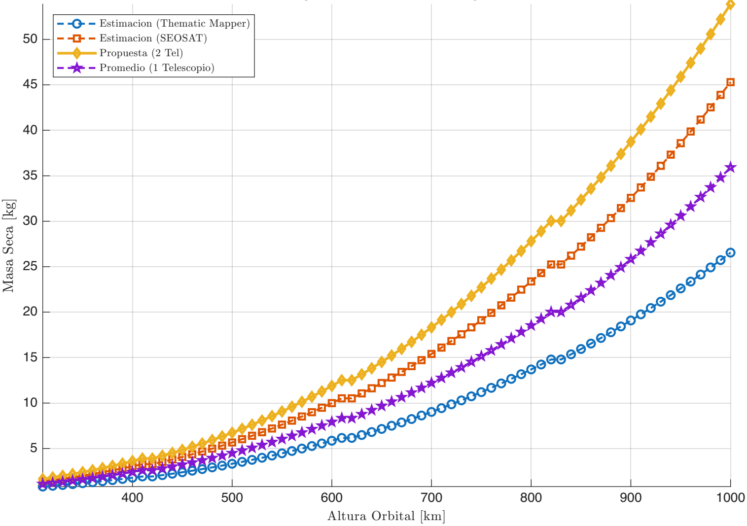
Comparativa de Masa Seca vs. Altura Config: 1 Sat, 2 Tel, Det 2, Cassegrain
